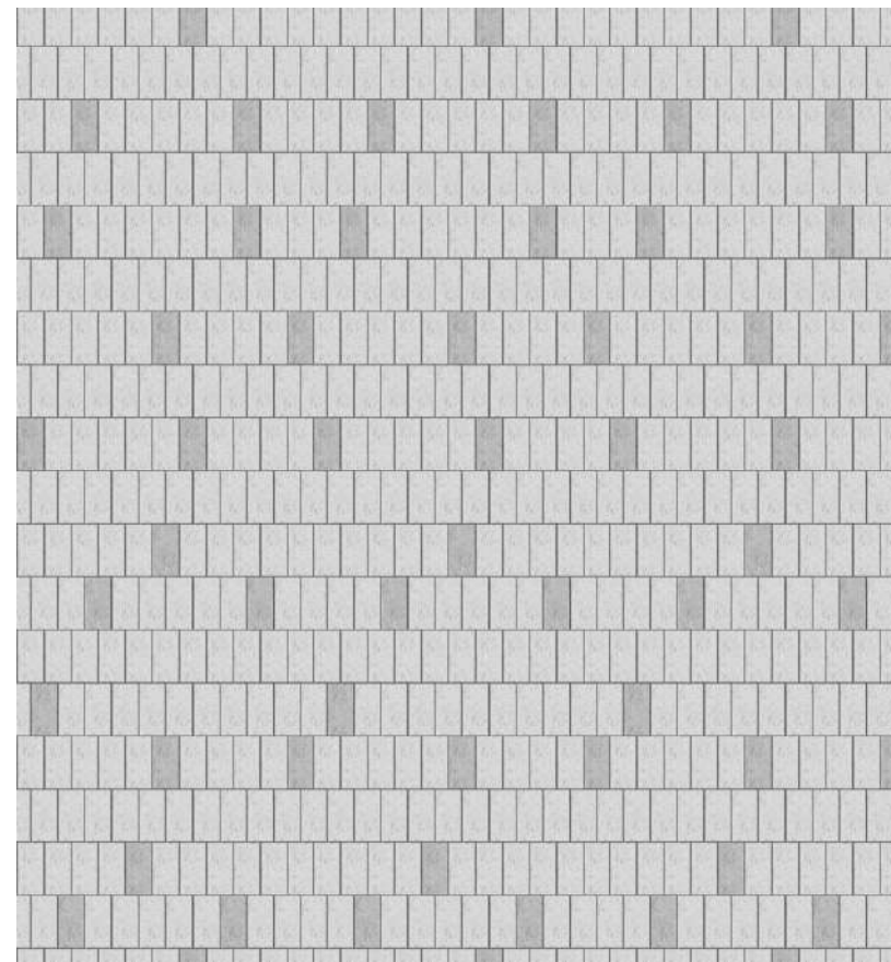
Рисунок мощения на основных маршрутах
